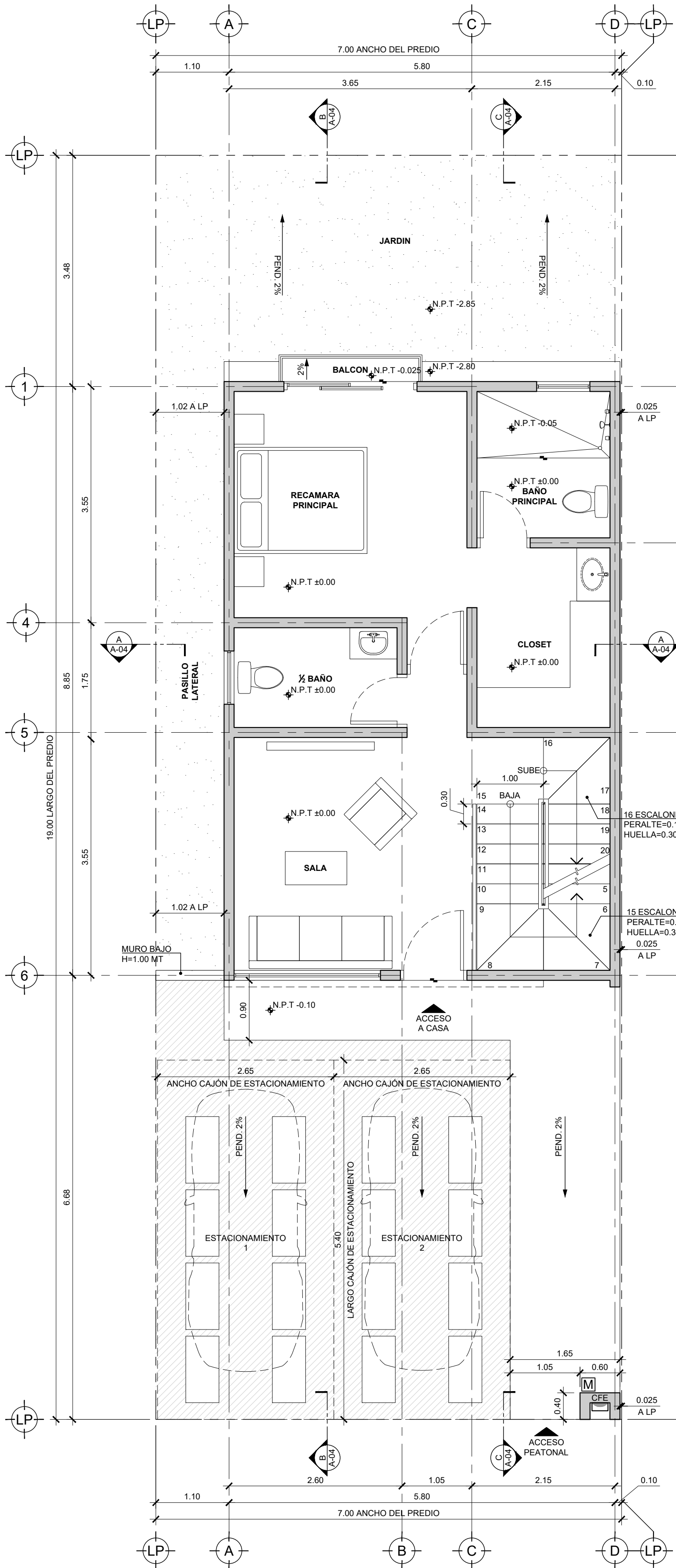
PLANTA BAJA ESC 1:50
