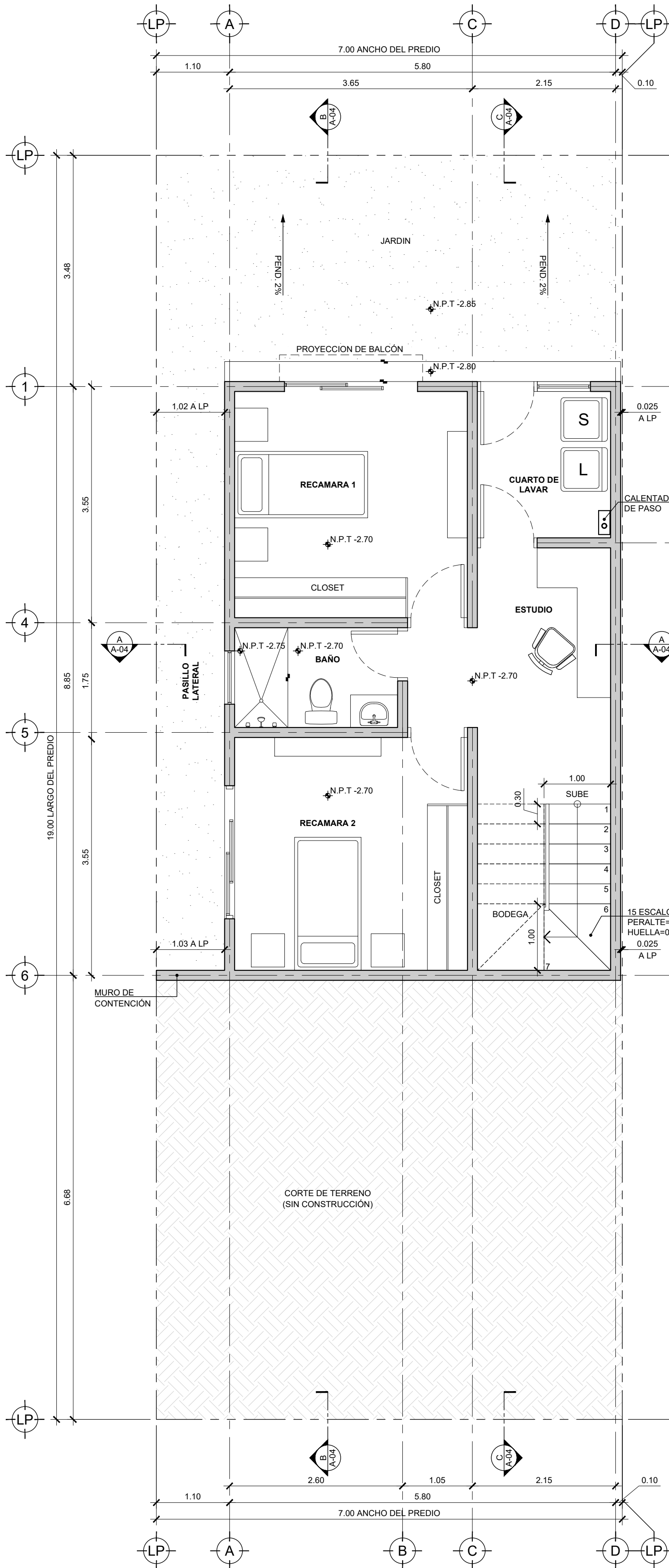
PLANTA NIVEL -1 ESC 1:50
